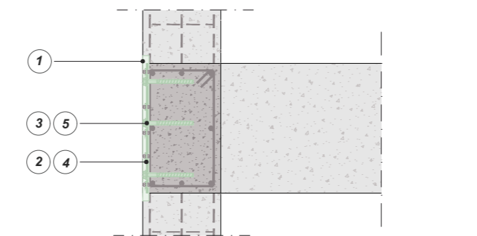
SEZIONE A-A' RINFORZO DEL NODO TRAVE PILASTRO A 2 VIE (D'ANGOLO) MEDIANTE SISTEMA STEEL COMBO
