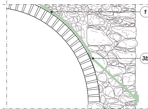
SEZIONE C-C' ANCORAGGIO PASSANTE PER I SISTEMI DI RINFORZO CON FASCE DI GEOSTEEL
