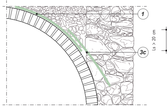
SEZIONE C-C' ANCORAGGIO CON DIATONI PER I SISTEMI DI RINFORZO CON RETE DIFFUSA GEOSTEEL GRID 200/400 O RINFORZO ARV 100
