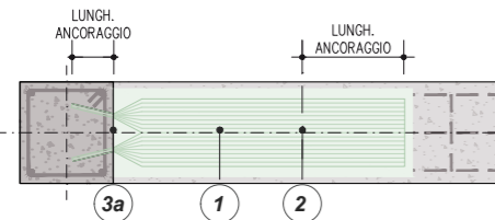
PIANTA A - A' RINFORZO A FLESSIONE DELLA TRAVE MEDIANTE PLACCAGGIO ESTRADOSSALE
