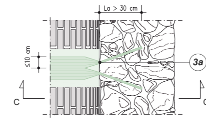
PIANTA ANCORAGGIO CIECO PER I SISTEMI DI RINFORZO CON FASCE DI GEOSTEEL
