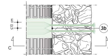
PIANTA ANCORAGGIO PASSANTE PER I SISTEMI DI RINFORZO CON FASCE DI GEOSTEEL
