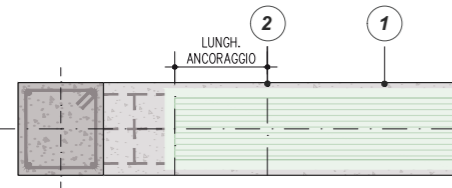
PIANTA B - B' RINFORZO A FLESSIONE DELLA TRAVE MEDIANTE PLACCAGGIO INTRADOSSALE
