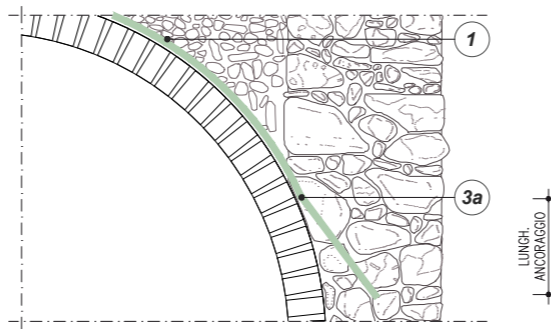
SEZIONE C-C' ANCORAGGIO CIECO PER I SISTEMI DI RINFORZO CON FASCE DI GEOSTEEL
