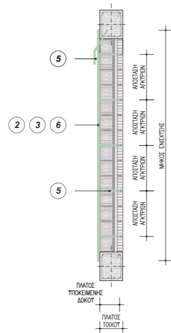
ΤΟΜΗ Α - Α' ΜΟΝΟΠΛΕΥΡΗ ΕΝΙΣΧΥΣΗ ΤΗΣ ΤΟΙΧΟΠΟΙΪΑΣ ΠΛΗΡΩΣΗΣ ΜΕ ΧΡΗΣΗ GEO GRID 120 ΚΑΙ ΑΓΚΥΡΙΩΝ STEEL DRYFIX 10 - ΠΡΟΛΗΨΗ ΑΠΟΚΟΛΛΗΣΗΣ
