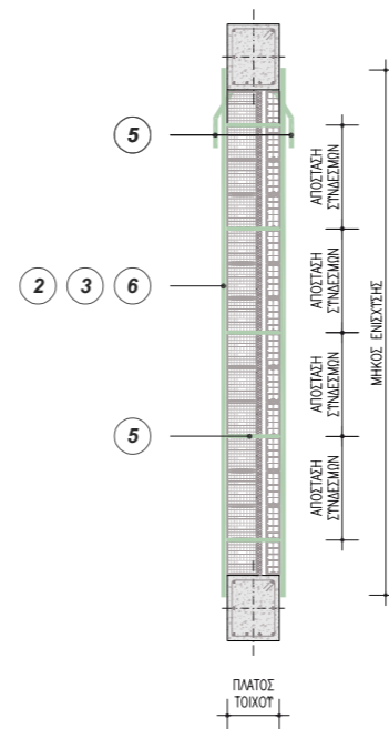
ΤΟΜΗ Α - Α' ΑΜΦΙΠΛΕΥΡΗ ΕΝΙΣΧΥΣΗ ΤΗΣ ΤΟΙΧΟΠΟΙΪΑΣ ΠΛΗΡΩΣΗΣ ΜΕ ΧΡΗΣΗ GEO GRID 120 ΚΑΙ ΑΓΚΥΡΙΩΝ STEEL DRYFIX 10 - ΠΡΟΛΗΨΗ ΑΠΟΚΟΛΛΗΣΗΣ
