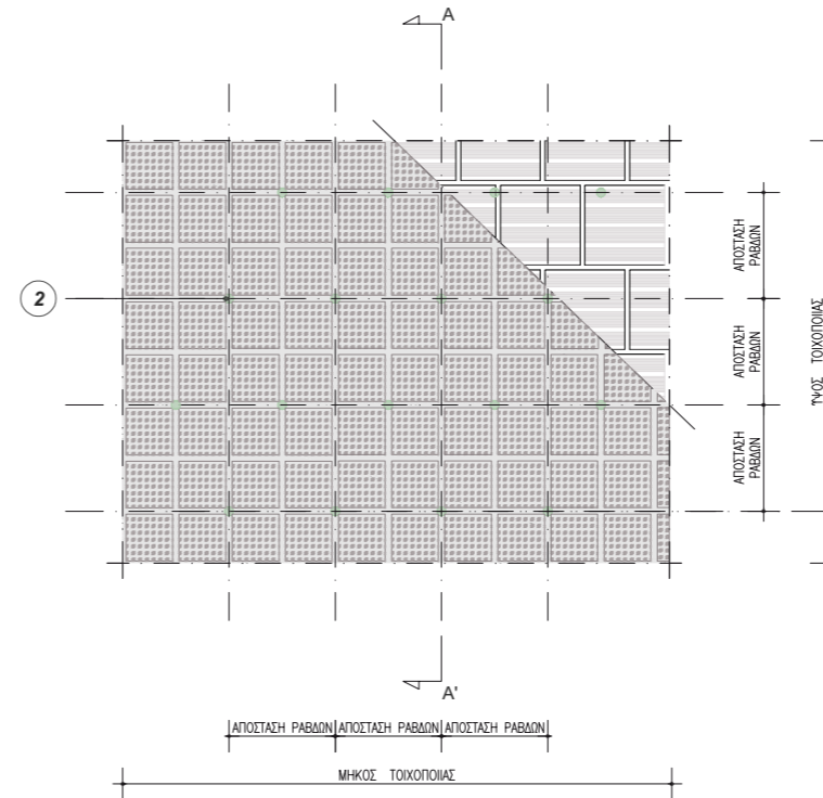
ΟΨΗ ΣΤΕΡΕΩΣΗ ΜΗ ΦΕΡΟΝΤΩΝ ΣΤΟΙΧΕΙΩΝ Ή ΣΤΟΙΧΕΙΩΝ ΠΡΟΣΟΨΗΣ ΜΕ ΤΟΠΟΘΕΤΗΣΗ ΑΓΚΥΡΙΩΝ ΥΨΗΛΗΣ ΣΥΝΑΦΕΙΑΣ STEEL DRYFIX® 10
