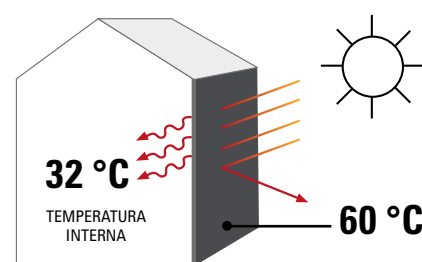
Stessa tinta con tecnologia tradizionale
