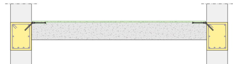
SEZIONE B - B' REALIZZAZIONE DI DIAFRAMMA DI PIANO MEDIANTE GETTO COLLABORANTE DI SISTEMA GEOLITE FRC E CONNETTORE PERIMETRALE STEEL CONNECT WALL
