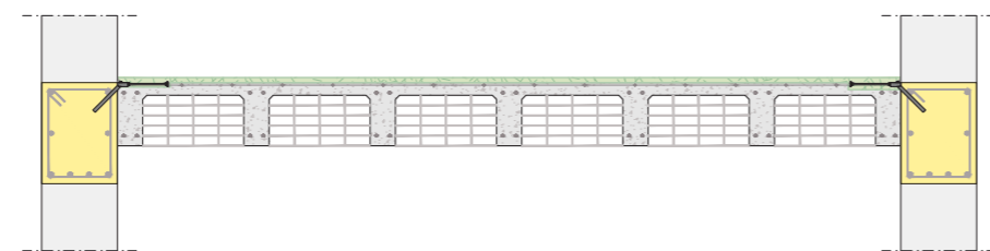
SEZIONE A - A' REALIZZAZIONE DI DIAFRAMMA DI PIANO MEDIANTE GETTO COLLABORANTE DI SISTEMA GEOLITE FRC E CONNETTORE PERIMETRALE STEEL CONNECT WALL
