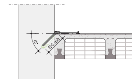
FASE I PREPARAZIONE DEL SUBSTRATO PER L'INSTALLAZIONE DEL CONNETTORE PERIMETRALE STEEL CONNECT WALL E SUCCESSIVO GETTO DEL SISTEMA GEOLITE FRC
