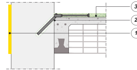
SOLUZIONE 1 CORDOLO IN TESSUTO DI FIBRA DI ACCIAIO GALVANIZZATO GEOSTEEL G600/G1200 ALLETTATO CON MALTA DI PURA CALCE IDARULICA NATURALE NHL3.5 GEOCALCE F ANTISISMICO + SISTEMA GEOLITE FRC E CONNETTORE PERIMETRALE STEEL CONNECT WALL
